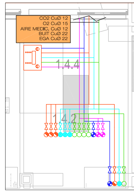
DETALL CONNEXIÓ DE GASOS MED. A GABINET 3
