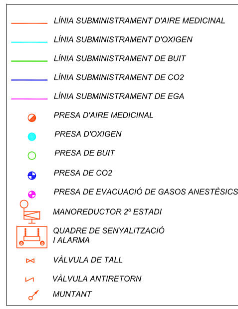
LLEGGENDA GASOS MEDICINALS
