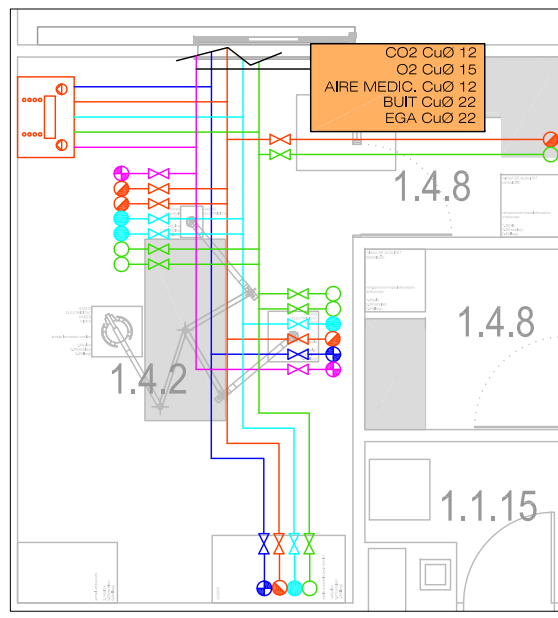
DETALL CONNEXIÓ DE GASOS MED. A GABINETS 1 I 2
